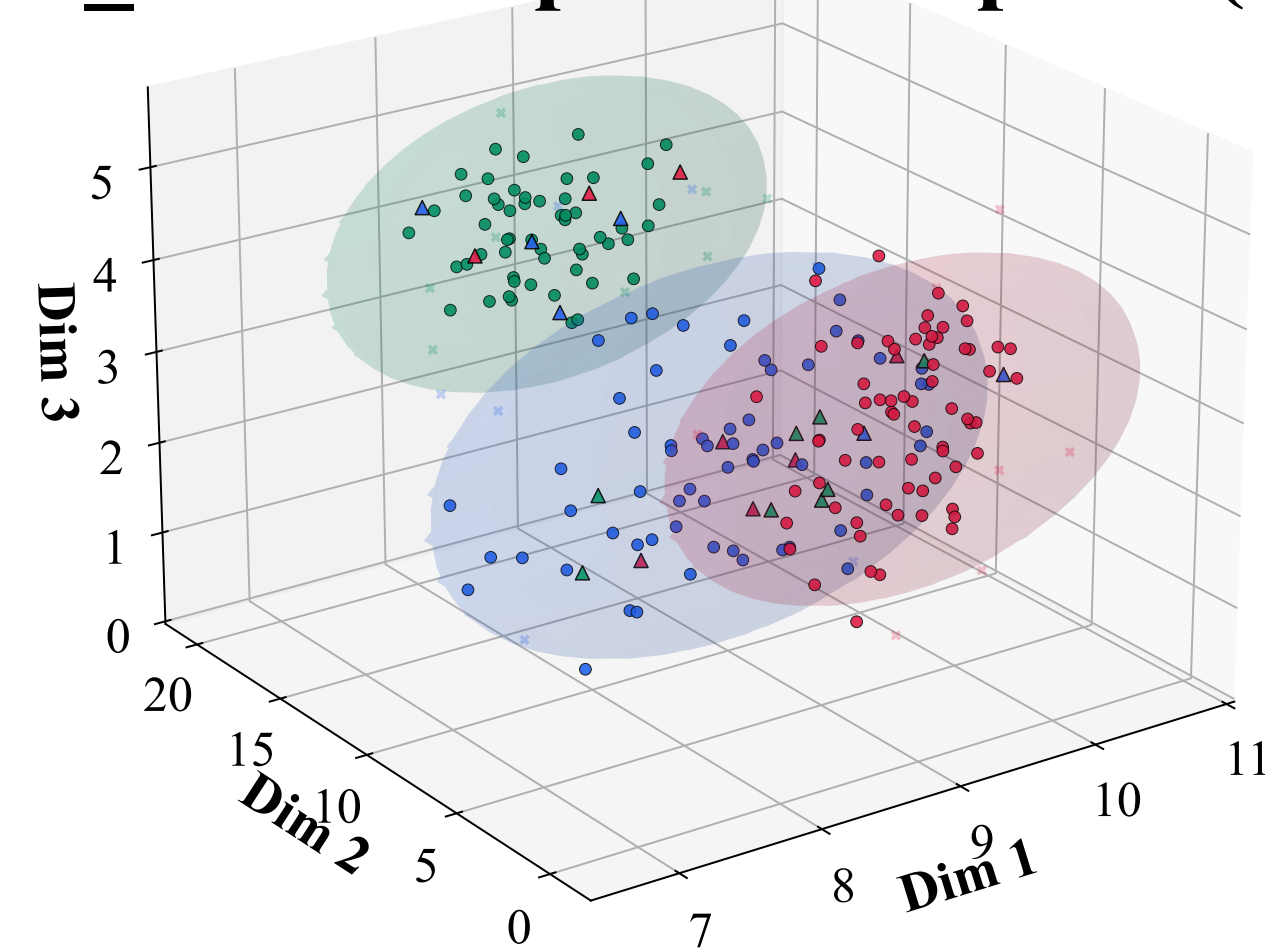
S_encoder Space — Explore (z=1)
